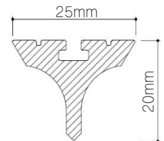
断面形状
